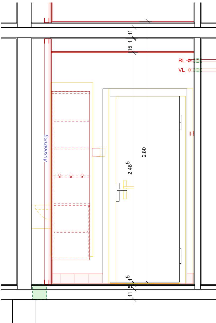
Ansicht C
