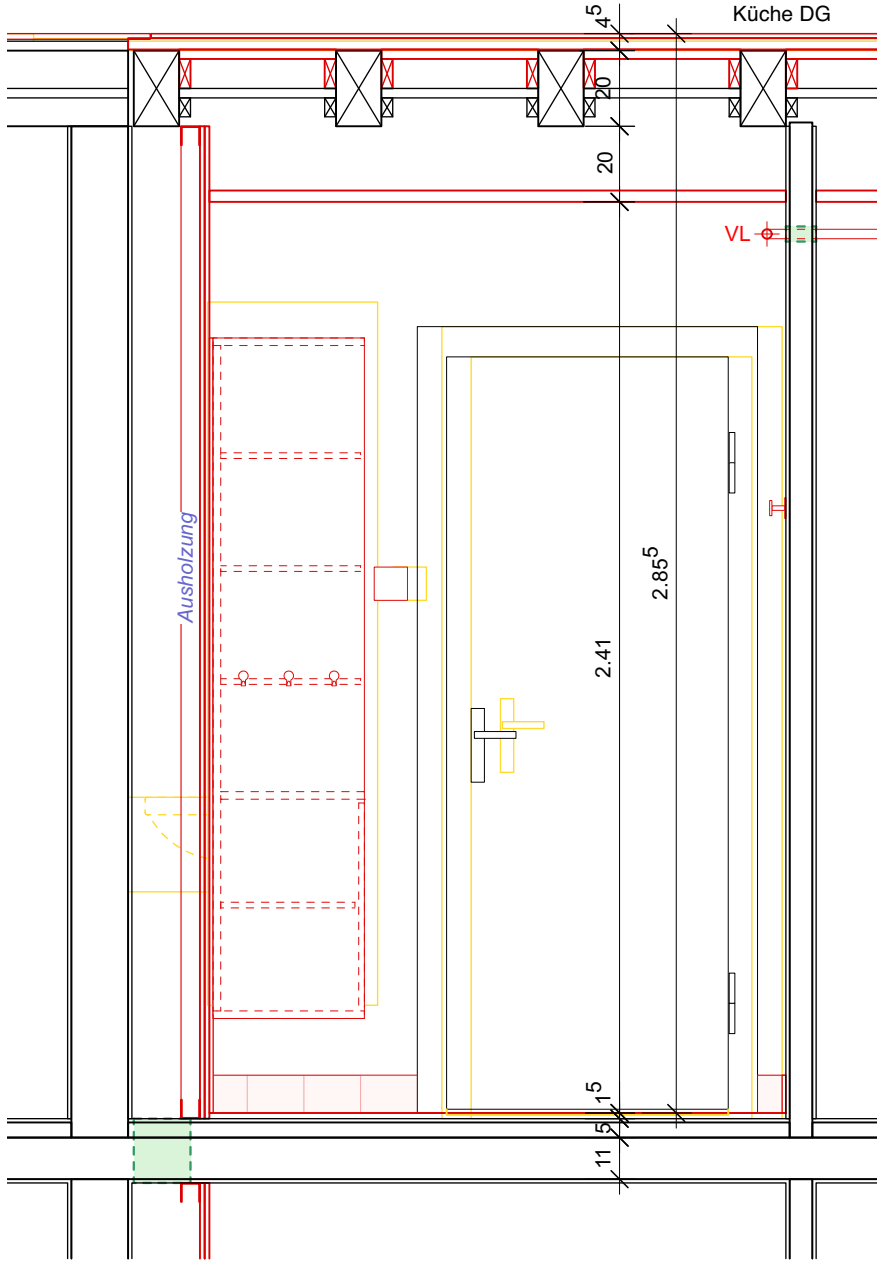
Ansicht C
