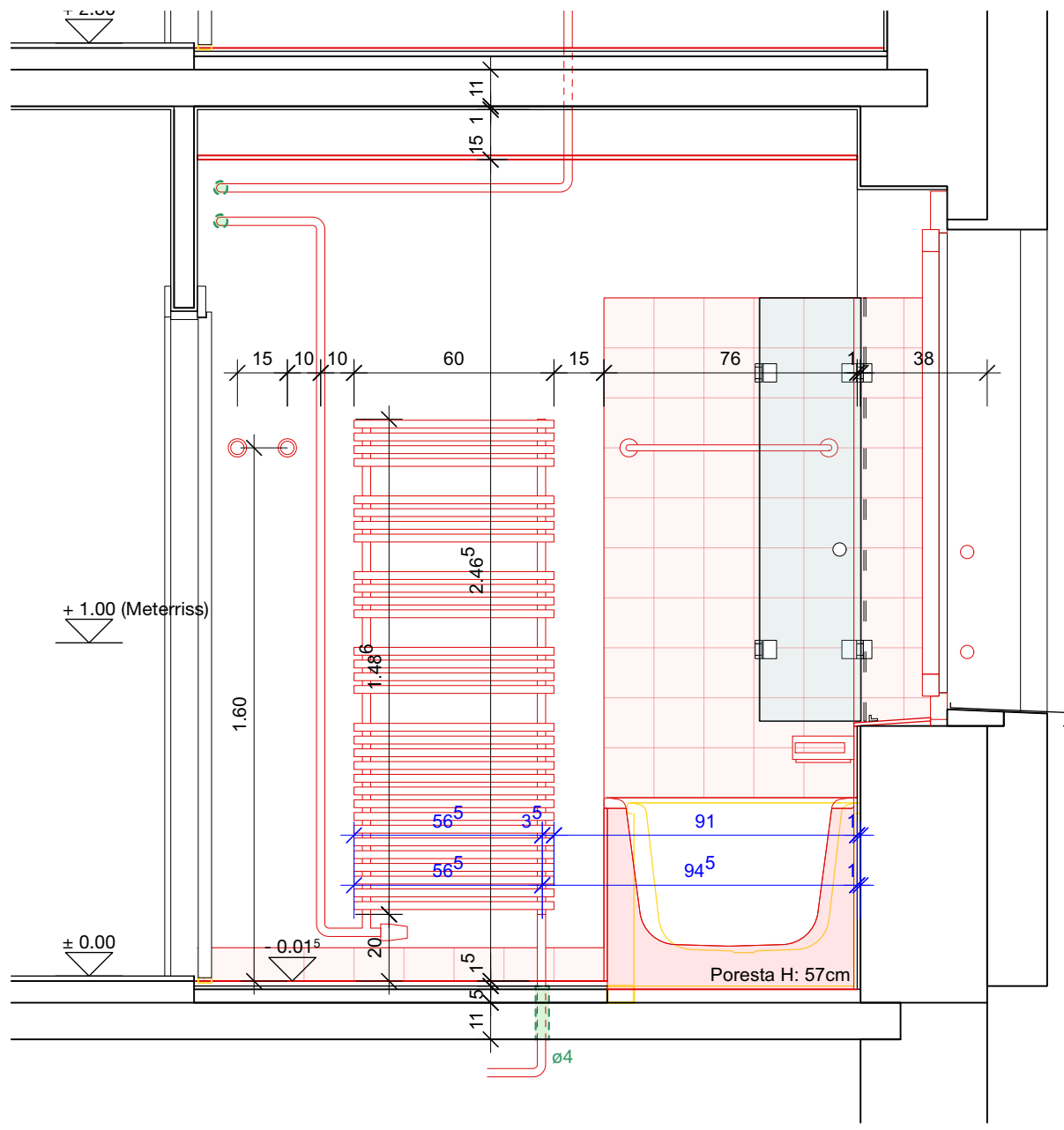
Ansicht D
