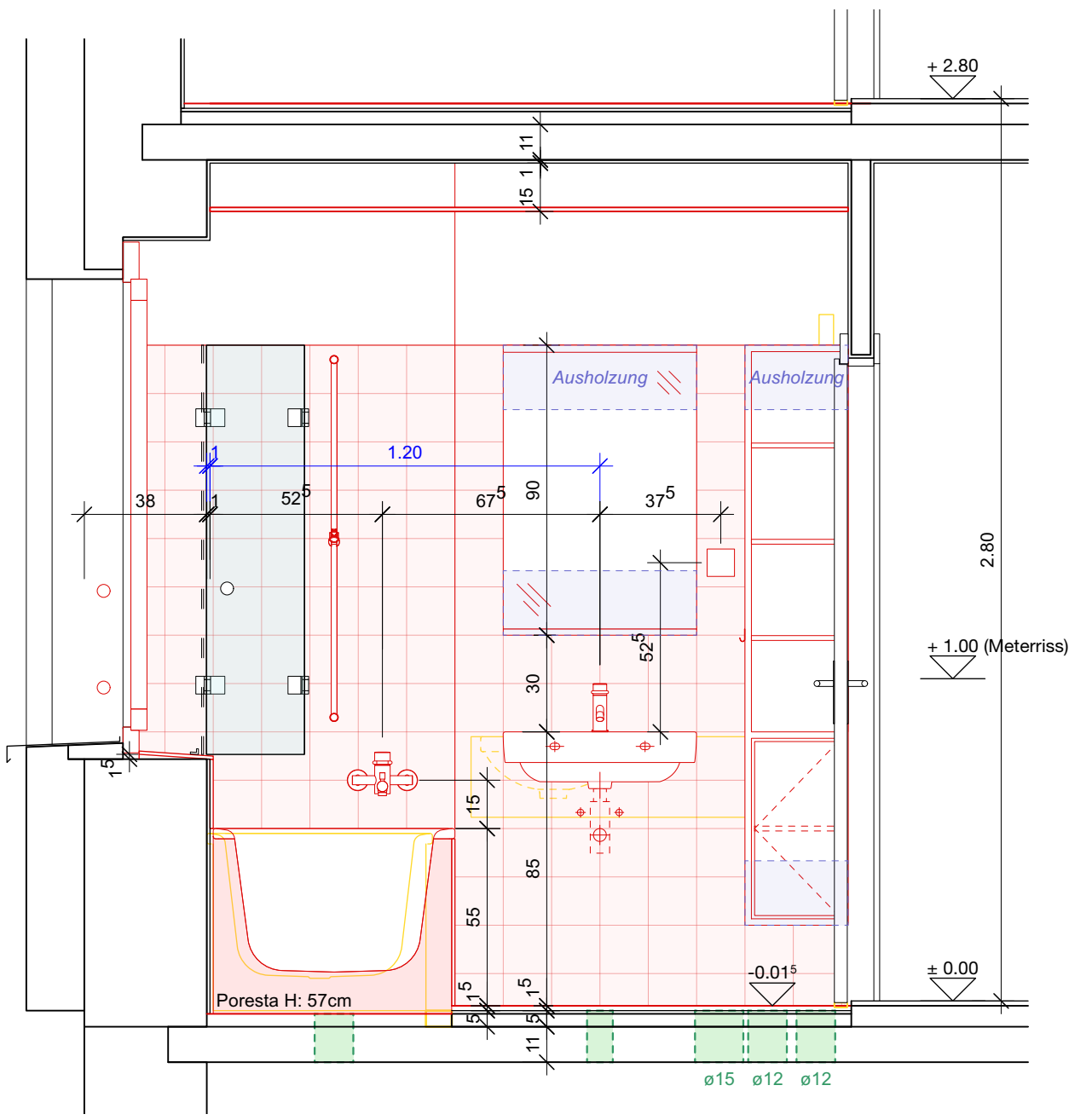
Ansicht B
