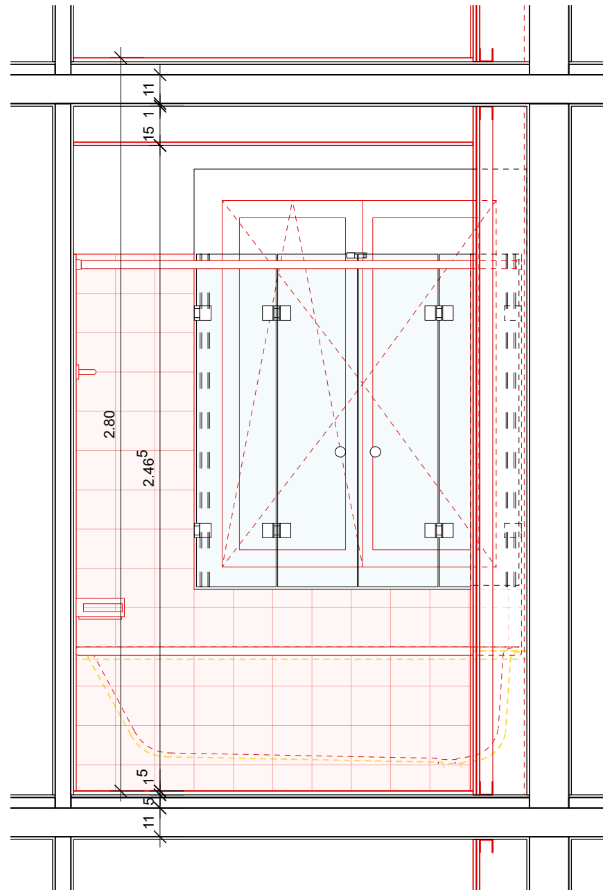
Ansicht A
