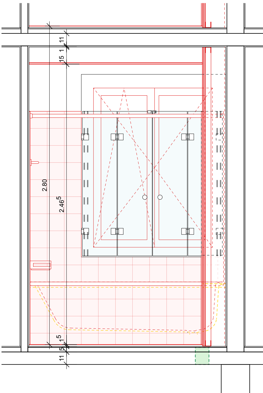
Ansicht A
