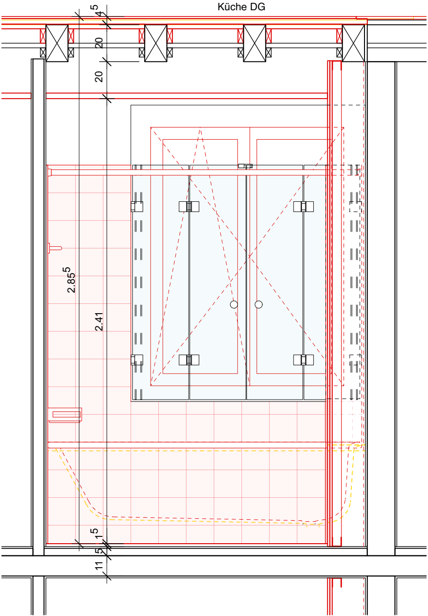
Ansicht A
