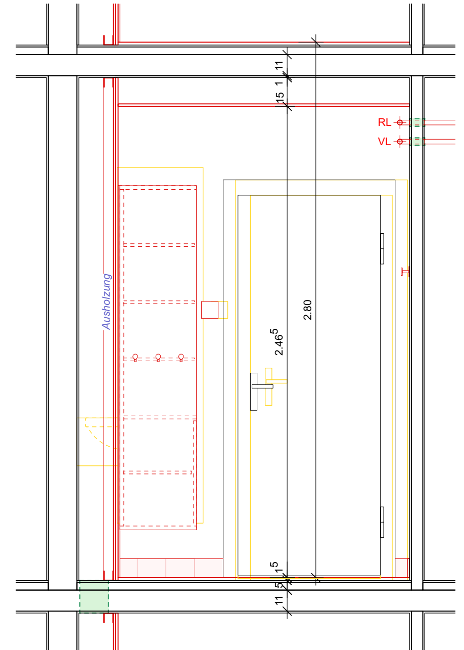
Ansicht C
