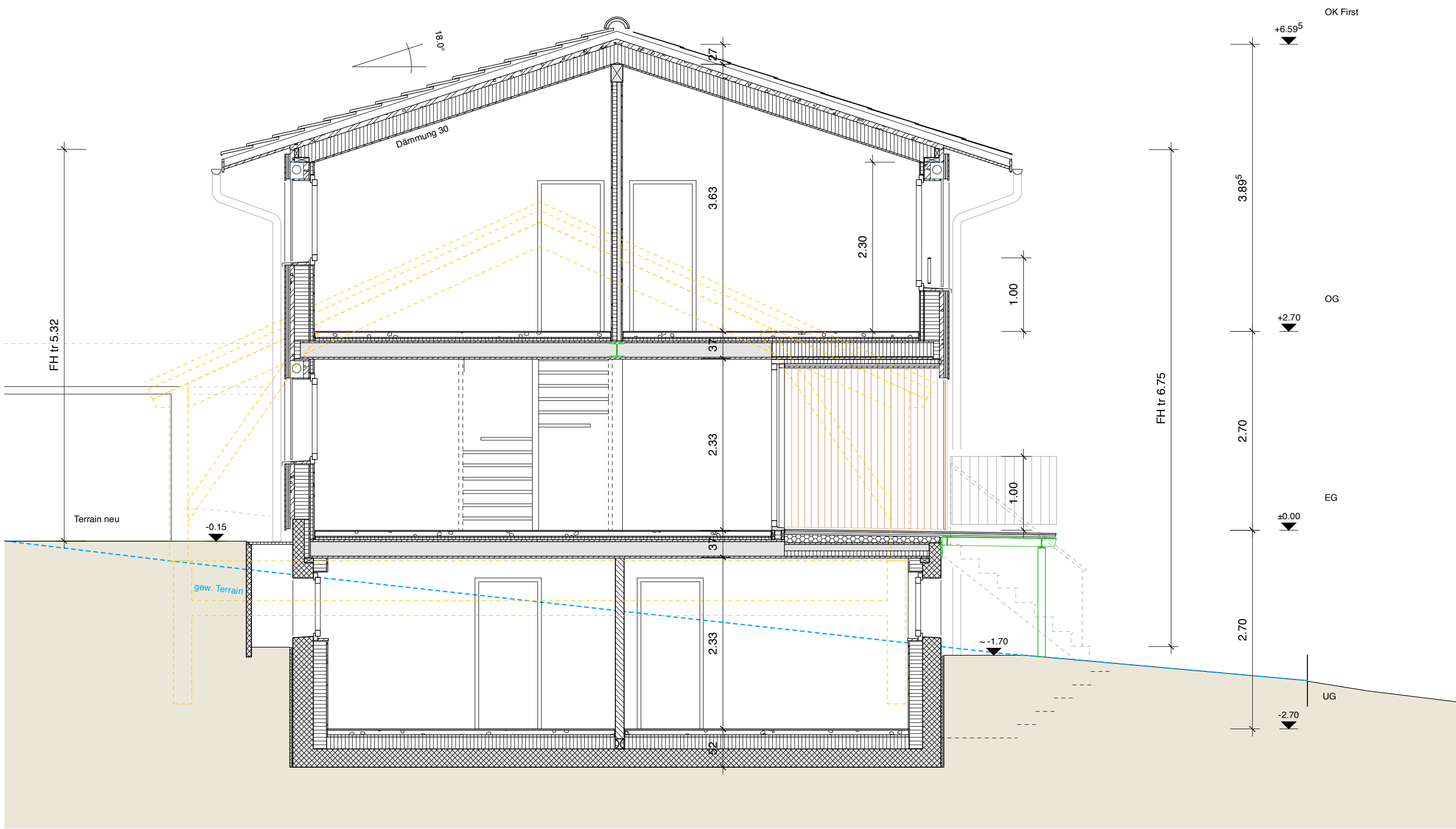
Schnitt A-A
