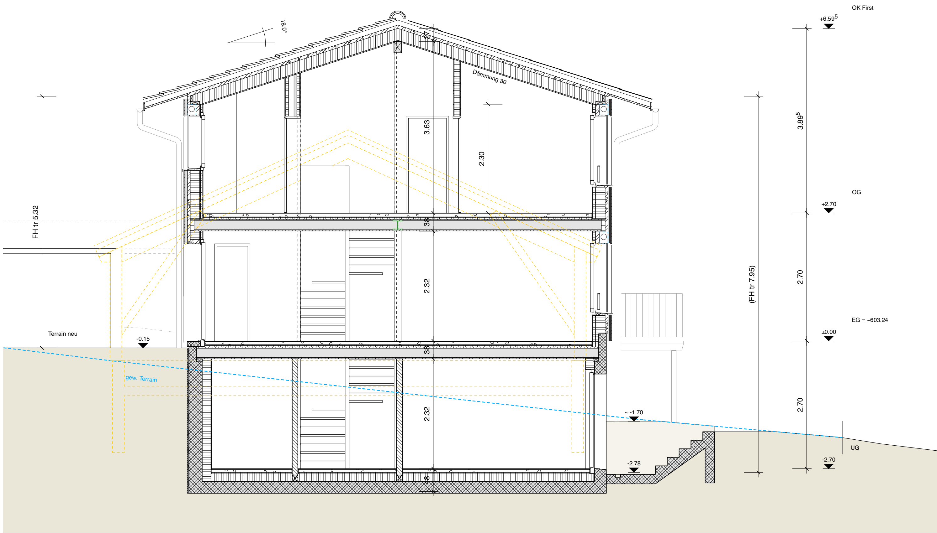
Schnitt B-B
